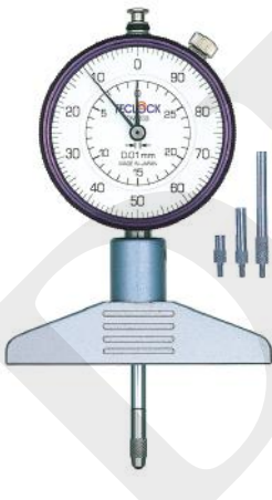
DM-233 継足の接続で最大 240mmまでの深さ測定が可能 ・継足5本付
