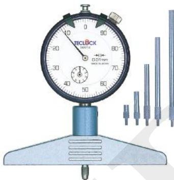
DM-210 使用用途の広い針状測定子タイプ
