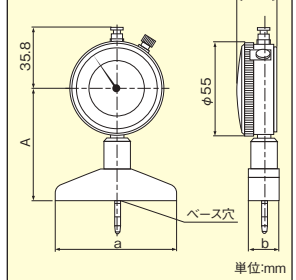
DM-234 継足の接続で最大240mmまでの 深さ測定が可能 ・継足5本付
