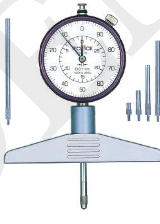
DM-234 継足の接続で最大240mmまでの 深さ測定が可能 ・継足5本付
