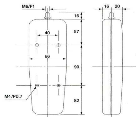
外型尺寸 Outline UNIT/mm
